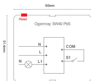
Фиг. 1. Схема на свързване
