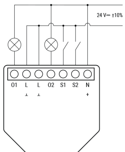
Zweikanal-Schaltmodus, Gleichstromversorgung
