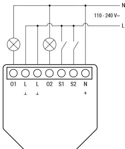
Zweikanal-Schaltmodus, Wechselstromversorgung
